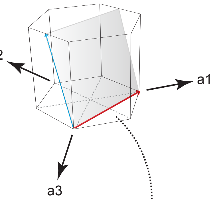
Tensile twin-2
